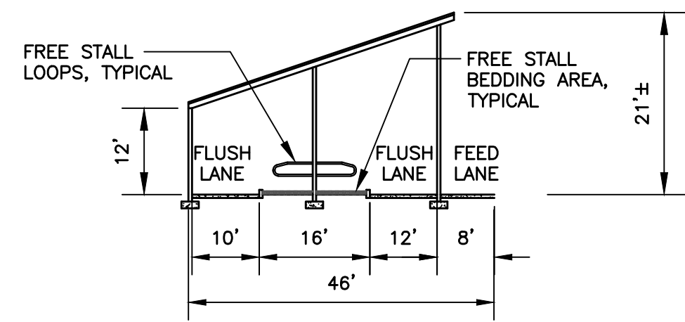
FREE STALL BARN END ELEVATION SCALE: 1" = 20'
