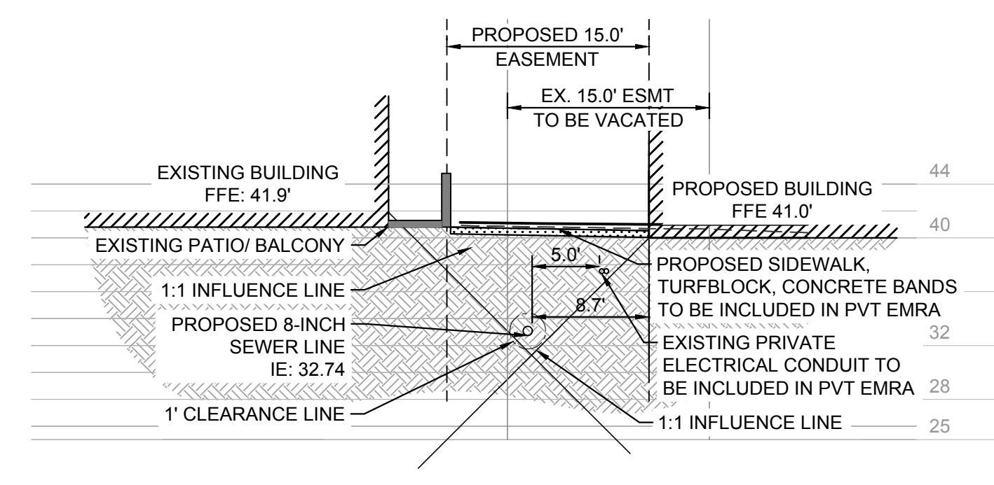
SEWER CROSS SECTION A-A SCALE: 1" = 10'
