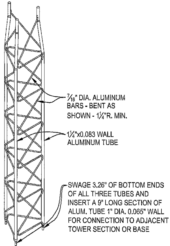
ISOMETRIC 3 SCALE: N.T.S.
