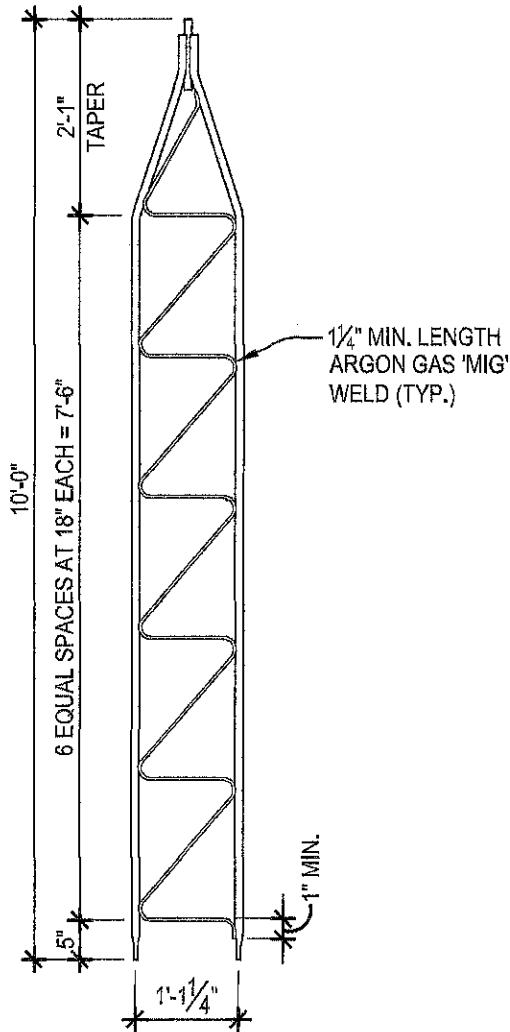
ELEVATION 2 SCALE: 1/2"=1'-0"
