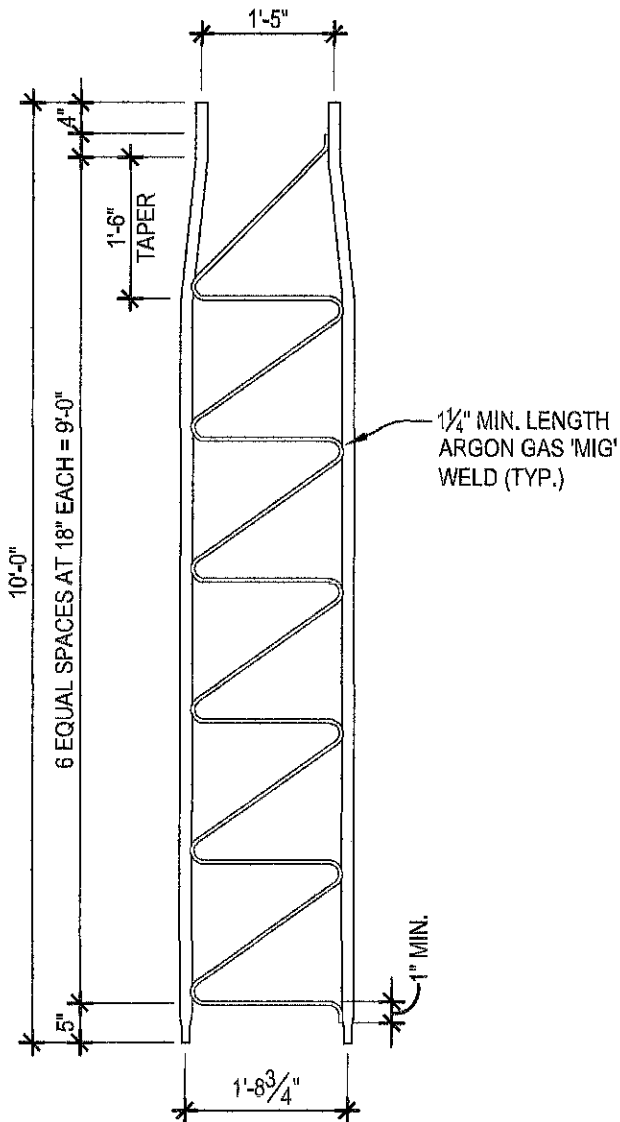
ELEVATION 2 SCALE: 1/2"=1'-0"
