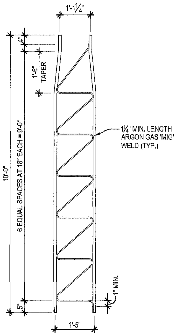
ELEVATION 2 SCALE: 1/2"=1'-0"
