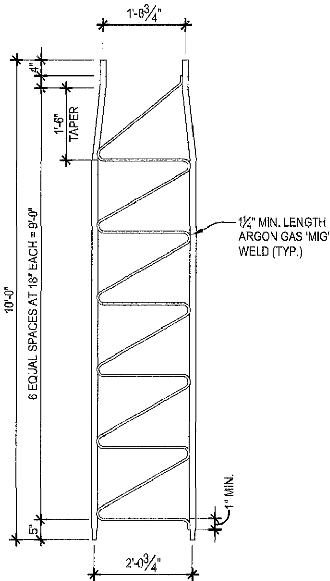
ELEVATION 2 SCALE: 1/2"=1'-0"
