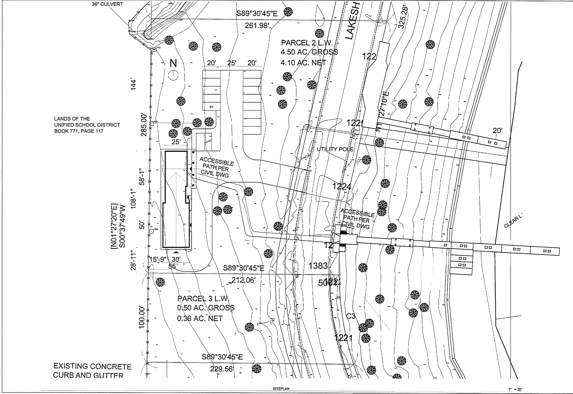
SITEPLAN
